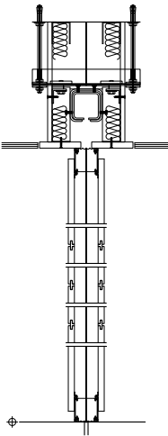
Compacts : les aiguillages interdépendants n'ont besoin que d'un espace axial minimal entre les paquets de rangement.
