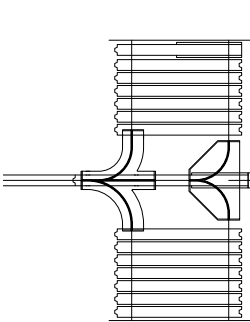
Codage mécanique : les éléments trouvent seuls leur voie dans la zone de rangement, ici en position parallèle droite.
