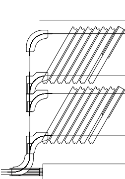
Compacts : les aiguillages interdépendants n'ont besoin que d'un espace axial minimal entre les paquets de rangement.
